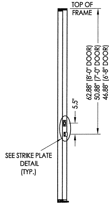
STRIKE JAMB
