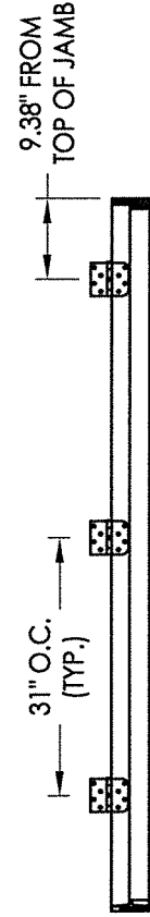
HINGE JAMB 7'-0" DOOR
