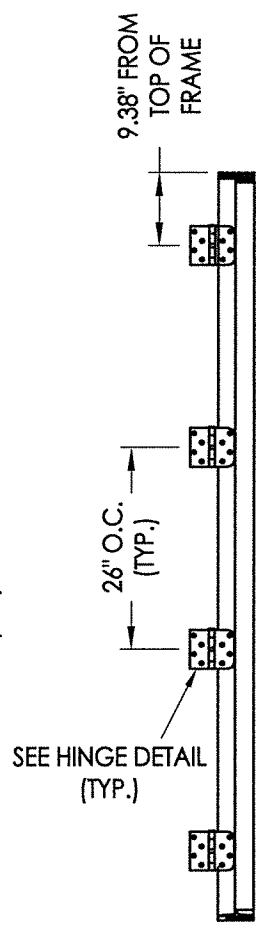
HINGE JAMB 8'-0" DOOR
