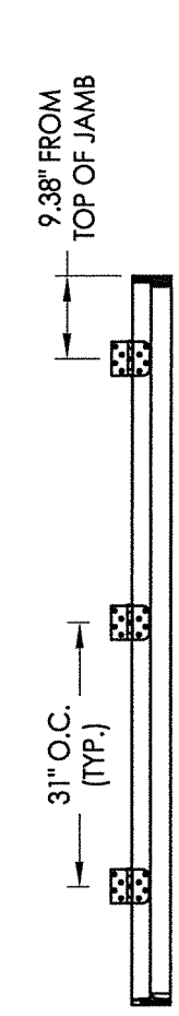
HINGE JAMB 7'-0" DOOR
