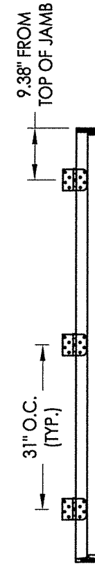
HINGE JAMB 6'-8" DOOR
